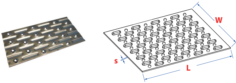
Spijkerplaat
