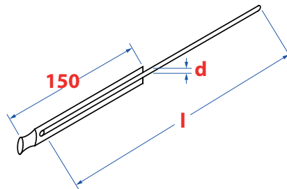
Slip tie Gleitanker
