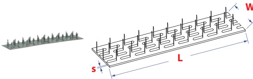
Multi-nagelplaat
